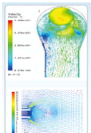
Моделирование поля течения при горении
