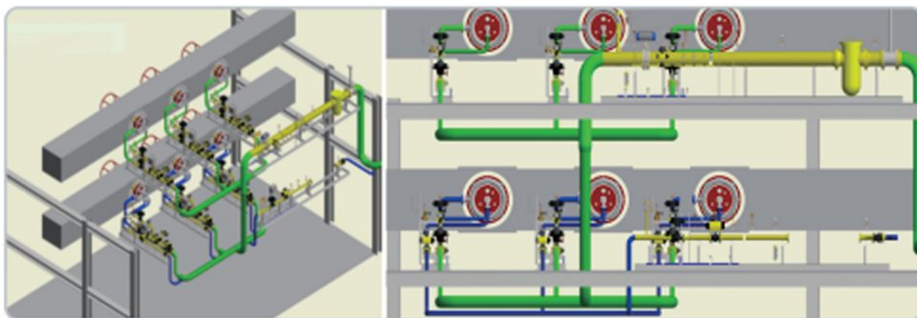
Компоновка блока группы клапанов горелки
